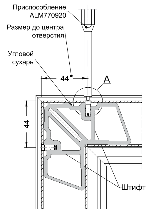
Схема установки штифтов
