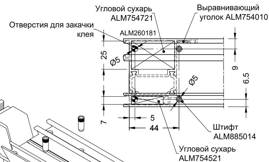
Приспособление: ALM770920
