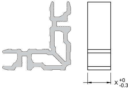
Допуск на ширину детали сухаря
